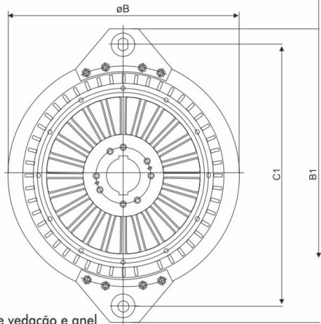
Disco de vedação e anel O'ring ( Não fazem parte do equipamento fornecido )
